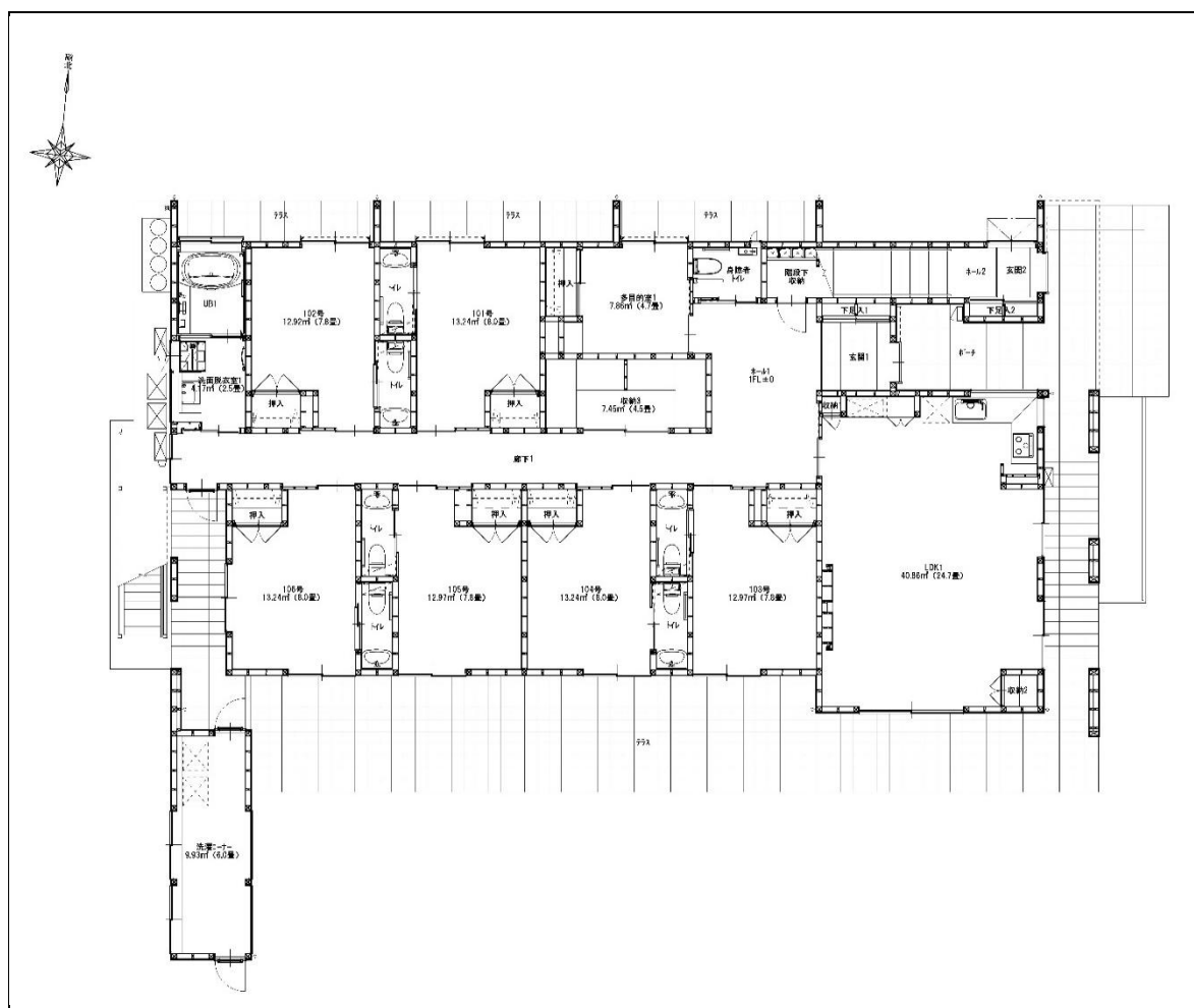
(建物 1 階 平面図)
