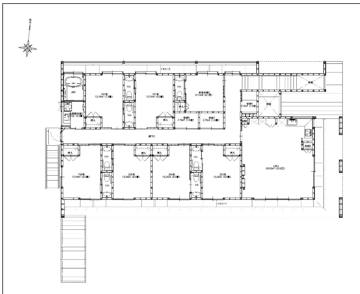
(建物2階 平面図)
